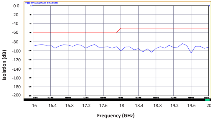
Isolation (16-20 GHz)
